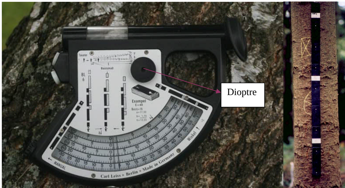
Figure 5 : Dendromètre Blume-Leiss et mire
