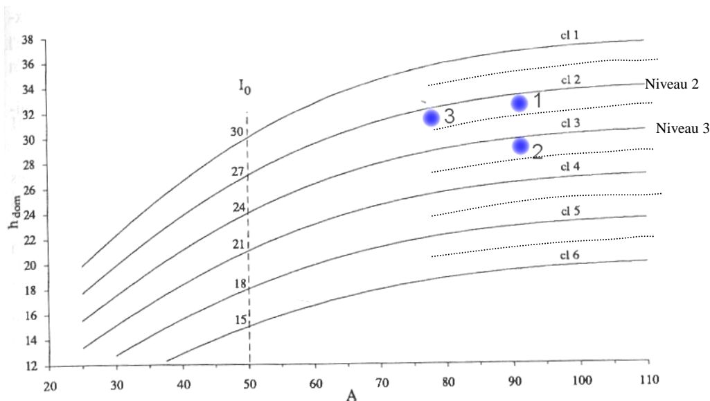
Figure 4 : Courbe de productivité établies pour l'épicéa commun dans les Ardennes belges ( Dagnelie P., Rondeux J. et al, 1988). I_0 = indice de productivité (site index) : hauteur dominante atteinte à 50 ans .
