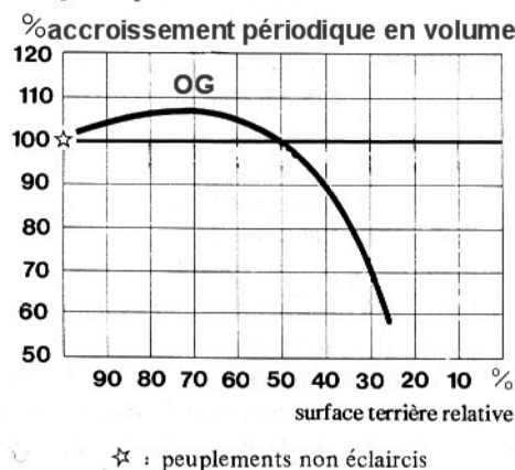
Figure 3 : Relation entre la productivité (mesurée par l'accroissement périodique en volume) et la densité (G) d'un peuplement ( Schutz J-Ph, 1990). OG représente la densité permettant d'obtenir la productivité optimale.
