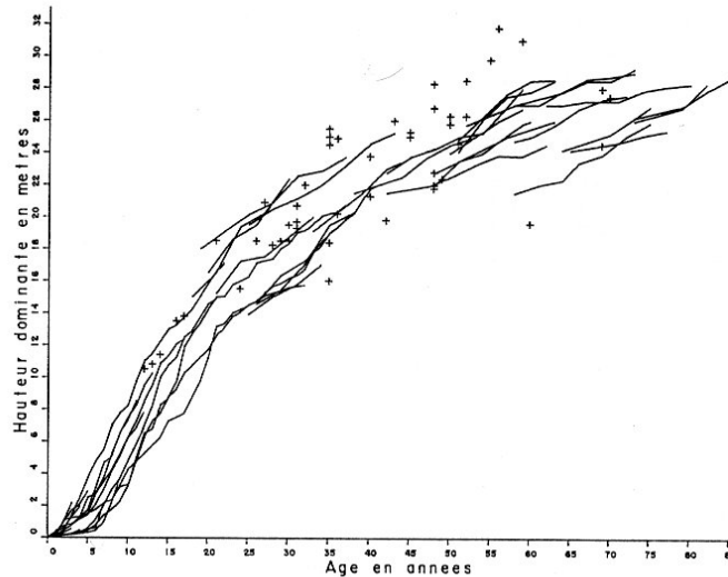
Figure 5 : Construction des courbes de productivité pour le frêne commun dans le Condroz belge ( Claessens H. et al., 1992). Les données proviennent de 27 placettes semi-permanentes, 48 placettes temporaires et 10 analyses de tiges.
