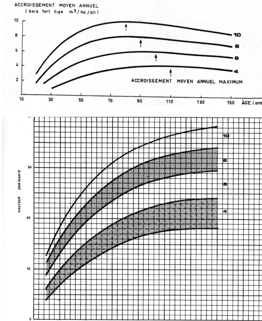
Figure 7 : Courbes de productivité anglaises (site index curves) valables pour le hêtre en Haute Normandie – hautes futaies équiennes ( Hamilton et Christie., 1971). Le chiffre en gras à droite représente la valeur du maximum de l'accroissement moyen annuel en volume.
